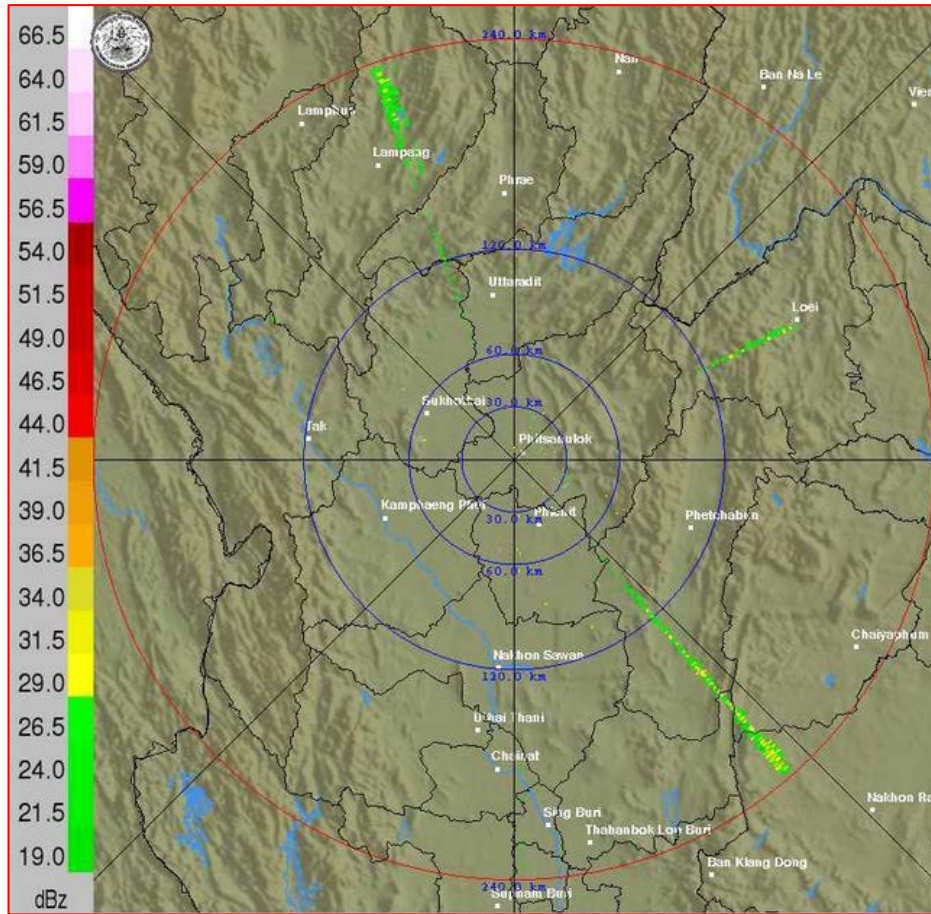
ภาพเรดาร์ตรวจอากาศ “พิชญ์โลก” ณ วันที่ 28 มกราคม 2563 (ที่มา : กรมอุตุนิยมวิทยา)
