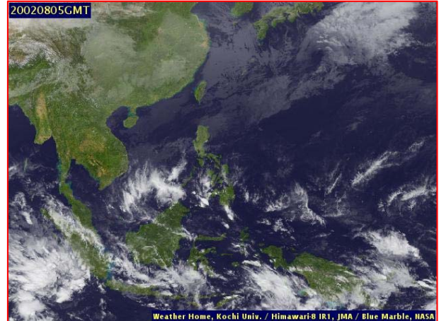
ภาพถ่ายดาวเทียม วันที่ ๘ ก.พ. ๒๕๖๓ เวลา ๑๒.๐๐ น.
