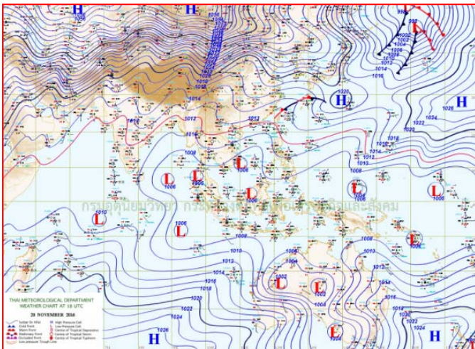
แผนที่อากาศ วันที่ ๒๑ พ.ย. ๒๕๕๙ เวลา ๐๑.๐๐ น.
