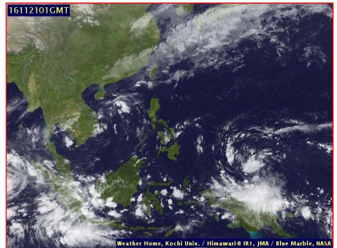
ภาพถ่ายจากดาวเทียม วันที่ ๒๑ พ.ย. ๒๕๕๙ เวลา ๐๘.๐๐ น.
