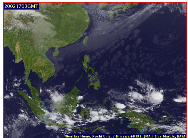
ภาพถ่ายดาวเทียม วันที่ ๑๗ ก.พ. ๒๕๖๓ เวลา ๑๐.๐๐ น.
