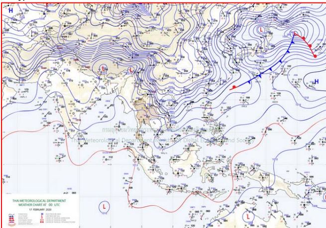
แผนที่อากาศ วันที่ ๑๗ ก.พ. ๒๕๖๓ เวลา ๑๒.๐๐ น.
