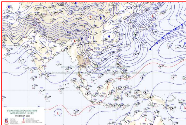
แผนที่อากาศ วันที่ ๑๘ ก.พ. ๒๕๖๓ เวลา ๐๑.๐๐ น.
