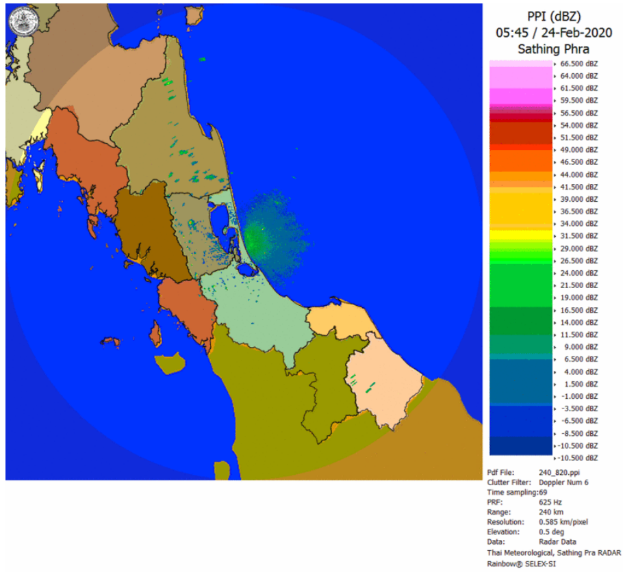
ภาพเรดาร์ตรวจอากาศ “สทิงพระ” ณ วันที่ 24 กุมภาพันธ์ 2563 (ที่มา : กรมอุตุนิยมวิทยา)
