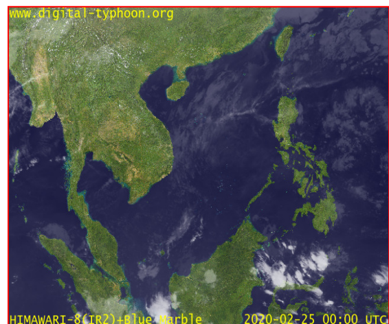
ภาพถ่ายจากดาวเทียม วันที่ 25 ก.พ. 2563
