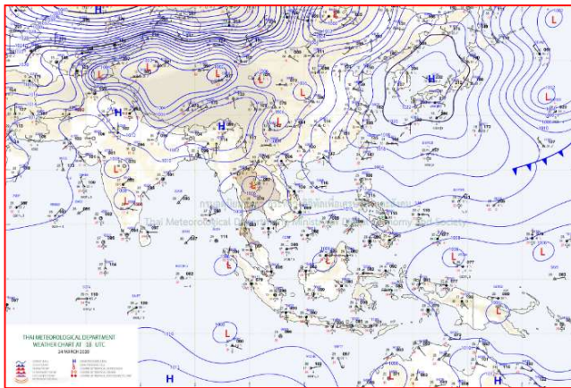
แผนที่อากาศ วันที่ ๒๕ มี.ค. ๒๕๖๓ เวลา ๐๑.๐๐ น.
