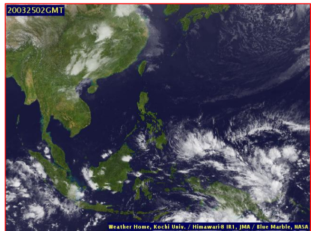
ภาพถ่ายดาวเทียม วันที่ ๒๕ มี.ค. ๒๕๖๓ เวลา ๐๙.๐๐ น.
