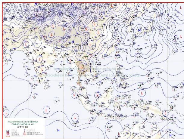
แผนที่อากาศ วันที่ ๒๕ มี.ค. ๒๕๖๓ เวลา ๐๗.๐๐ น.
