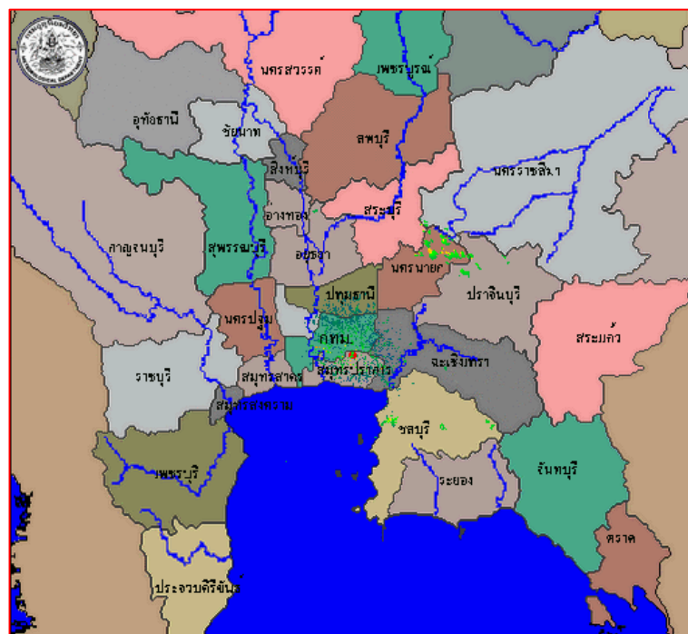
ภาพเรดาร์ตรวจอากาศ “สุวรรณภูมิ” ณ วันที่ 29 พฤศจิกายน 2559 (ที่มา : กรมอุตุนิยมวิทยา)
