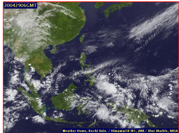
ภาพถ่ายดาวเทียม วันที่ ๒๙ เม.ย. ๒๕๖๓ เวลา ๑๓.๐๐ น.
