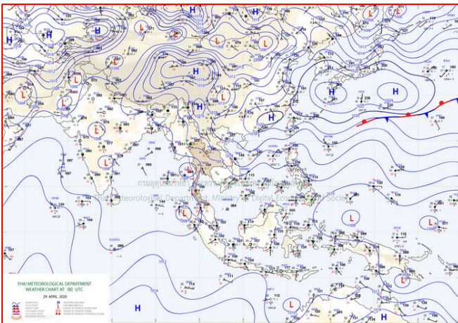
แผนที่อากาศ วันที่ ๒๙ เม.ย. ๒๕๖๓ เวลา ๐๗.๐๐ น.
