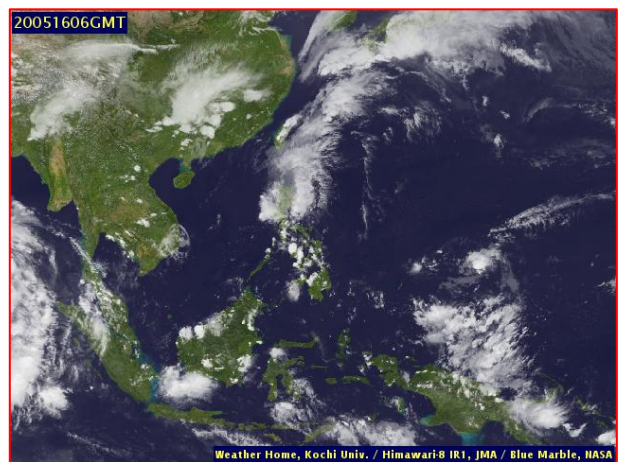
ภาพถ่ายดาวเทียม วันที่ ๑๖ พ.ค. ๒๕๖๓ เวลา ๑๓.๐๐ น.
