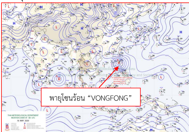
แผนที่อากาศ วันที่ ๑๖ พ.ค. ๒๕๖๓ เวลา ๐๗.๐๐ น.
