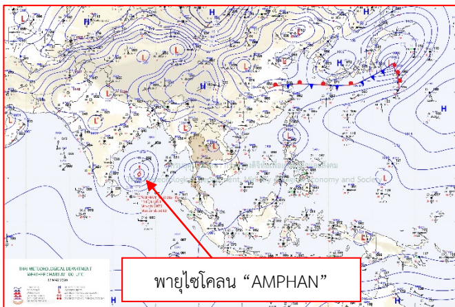
แผนที่อากาศ วันที่ ๑๘ พ.ค. ๒๕๖๓ เวลา ๐๑.๐๐ น.
