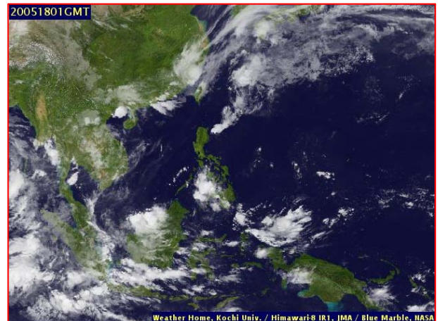
ภาพถ่ายดาวเทียม วันที่ ๑๘ พ.ค. ๒๕๖๓ เวลา ๐๘.๐๐ น.
