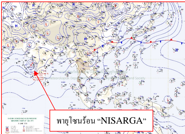
แผนที่อากาศ วันที่ ๓ มิ.ย. ๒๕๖๓ เวลา ๐๗.๐๐ น.
