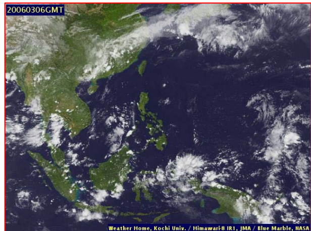
ภาพถ่ายดาวเทียม วันที่ ๓ มิ.ย. ๒๕๖๓ เวลา ๑๓.๐๐ น.
