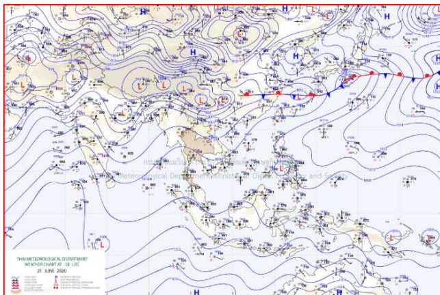
แผนที่อากาศ วันที่ ๒๒ มิ.ย. ๒๕๖๓ เวลา ๐๑.๐๐ น.
