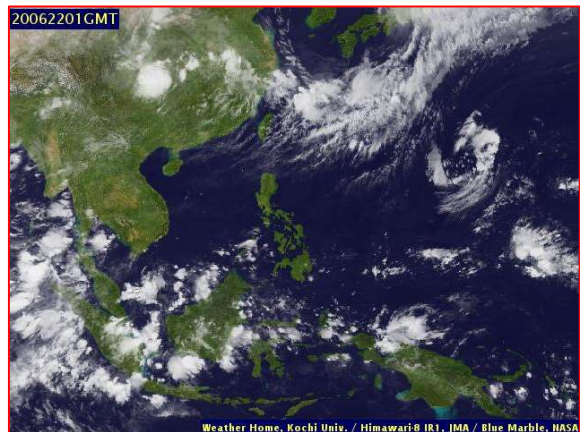
ภาพถ่ายดาวเทียม วันที่ ๒๒ มิ.ย. ๒๕๖๓ เวลา ๐๘.๐๐ น.
