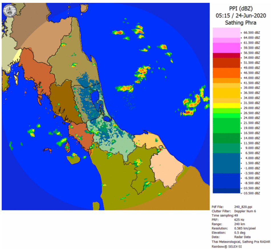
ภาพเรดาร์ตรวจอากาศ “สathingพระ” ณ วันที่ 24 มิถุนายน 2563 (ที่มา : กรมอุตุนิยมวิทยา)
