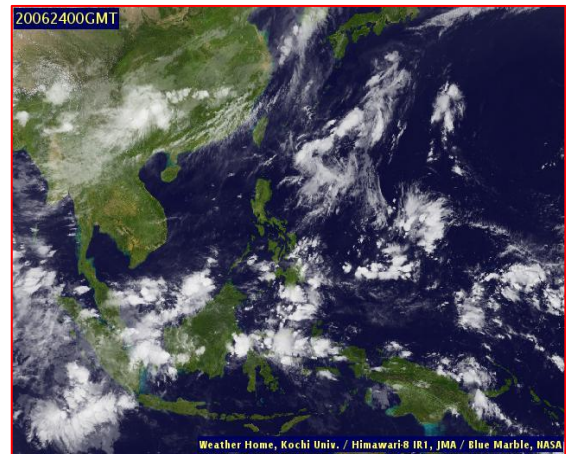
ภาพถ่ายจากดาวเทียม วันที่ 24 มิ.ย. 2563
