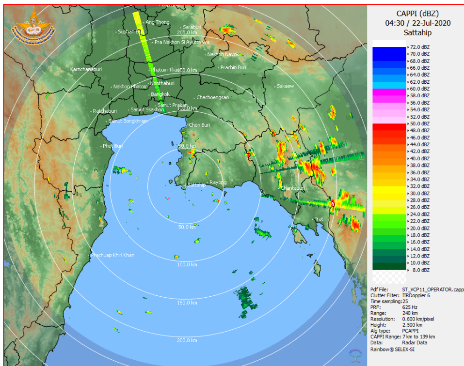
ภาพเรดาร์ตรวจอากาศ “สถานีสัตหีบ” ณ วันที่ 22 กรกฎาคม 2563 เวลา 11.30 น. (ที่มา : กรมอุตุนิยมวิทยา)
