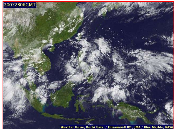
ภาพถ่ายดาวเทียม วันที่ ๒๘ ก.ค. ๒๕๖๓ เวลา ๑๓.๐๐ น.
