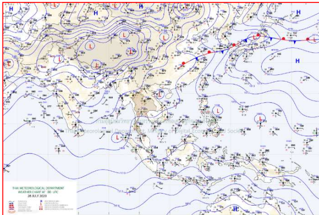
แผนที่อากาศ วันที่ ๒๘ ก.ค. ๒๕๖๓ เวลา ๐๗.๐๐ น.
