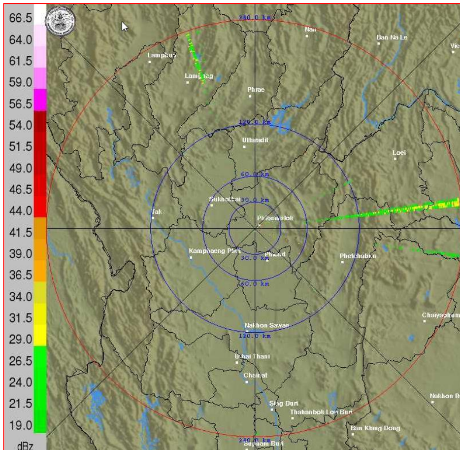
ภาพเรดาร์ตรวจอากาศ “พิษณุโลก” ณ วันที่ 31 กรกฎาคม 2563 (ที่มา : กรมอุตุนิยมวิทยา)
