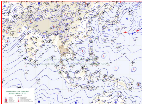
แผนที่อากาศ วันที่ 31 ก.ค. 2563 เวลา 07.00 น.
