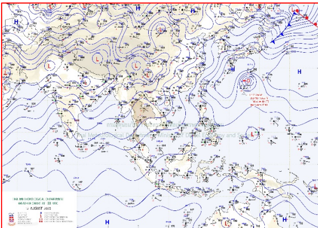
แผนที่อากาศ วันที่ ๑๒ ส.ค. ๒๕๖๓ เวลา ๐๗.๐๐ น.
