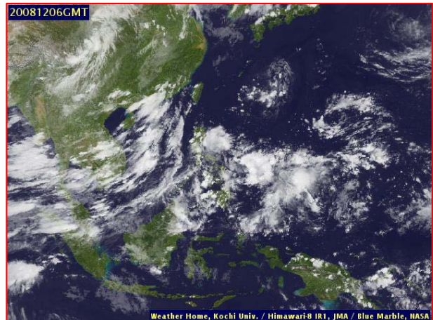
ภาพถ่ายดาวเทียม วันที่ ๑๒ ส.ค. ๒๕๖๓ เวลา ๑๓.๐๐ น.
