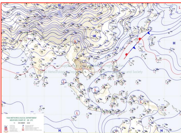
แผนที่อากาศ วันที่ ๑๒ ธ.ค. ๒๕๖๓ เวลา ๐๑.๐๐ น.
