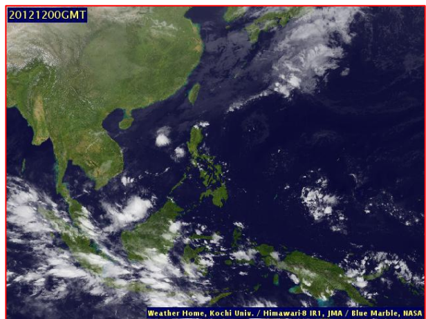
ภาพถ่ายดาวเทียม วันที่ ๑๒ ธ.ค. ๒๕๖๓ เวลา ๐๗.๐๐ น.
