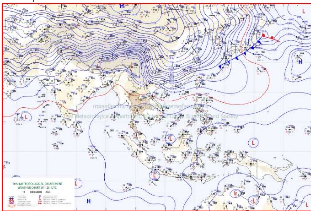
แผนที่อากาศ วันที่ ๑๔ ธ.ค. ๒๕๖๓ เวลา ๐๑.๐๐ น.
