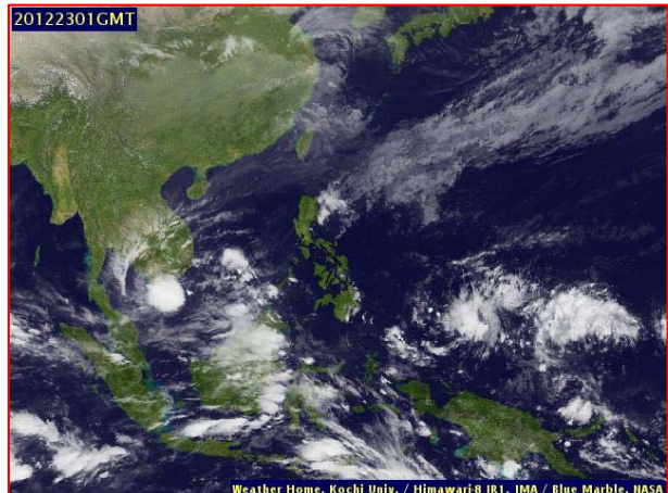
ภาพถ่ายดาวเทียม วันที่ ๒๓ ธ.ค. ๒๕๖๓ เวลา ๐๘.๐๐ น.
