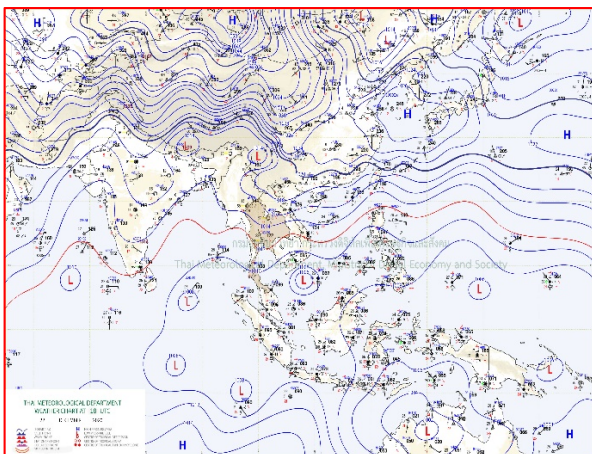
แผนที่อากาศ วันที่ ๒๓ ธ.ค. ๒๕๖๓ เวลา ๐๑.๐๐ น.
