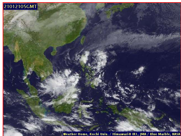
ภาพถ่ายดาวเทียม วันที่ ๒๑ ม.ค. ๒๕๖๔ เวลา ๑๒.๐๐ น.
