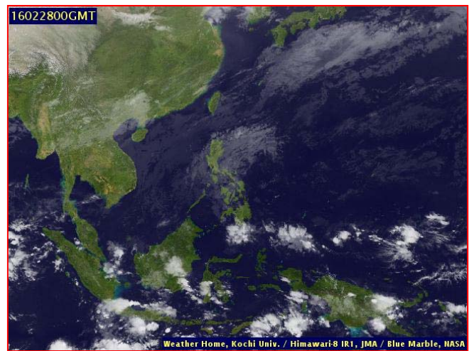
ภาพถ่ายจากดาวเทียม วันที่ ๒๘ ก.พ. ๒๕๕๙ เวลา ๐๗.๐๐ น.
