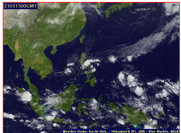
ภาพถ่ายดาวเทียม วันที่ ๑๕ มี.ค. ๒๕๖๔ เวลา ๐๗.๐๐ น.
