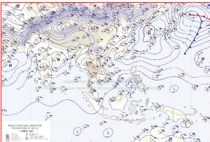
แผนที่อากาศ วันที่ ๑๕ มี.ค. ๒๕๖๔ เวลา ๐๑.๐๐ น.
