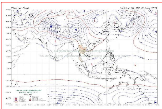
แผนที่อากาศ วันที่ ๒ พ.ค. ๒๕๖๔ เวลา ๐๑.๐๐ น.
