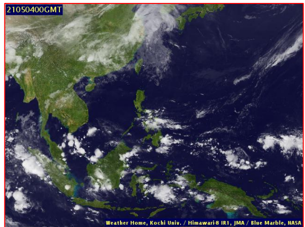
ภาพถ่ายดาวเทียม วันที่ ๔ พ.ค. ๒๕๖๔ เวลา ๐๗.๐๐ น.
