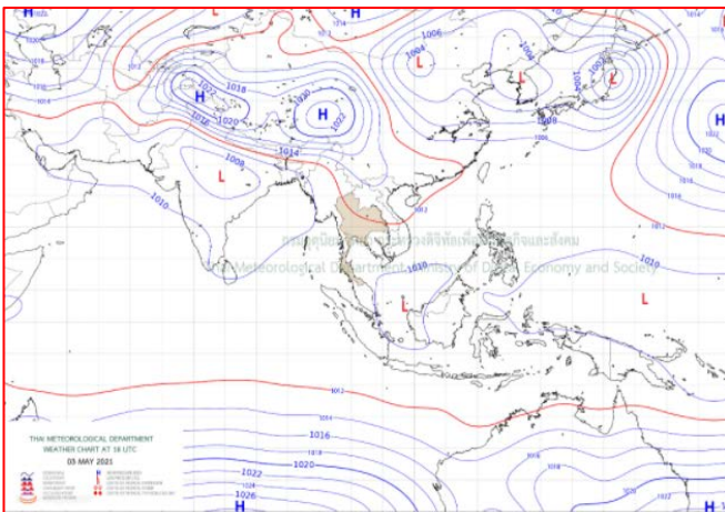
แผนที่อากาศ วันที่ ๔ พ.ค. ๒๕๖๔ เวลา ๐๑.๐๐ น.
