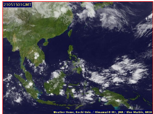
ภาพถ่ายดาวเทียม วันที่ ๑๕ พ.ค. ๒๕๖๔ เวลา ๐๘.๐๐ น.
