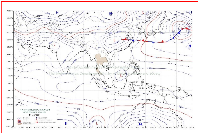
แผนที่อากาศ วันที่ ๑๕ พ.ค. ๒๕๖๔ เวลา ๐๑.๐๐ น.
