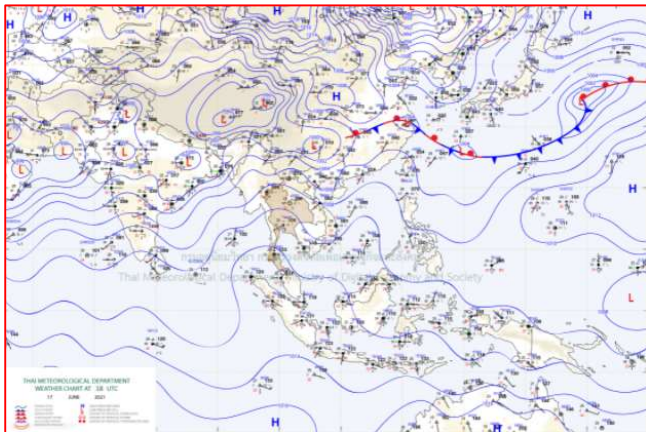
แผนที่อากาศ วันที่ ๑๘ มิ.ย. ๒๕๖๔ เวลา ๐๑.๐๐ น.
