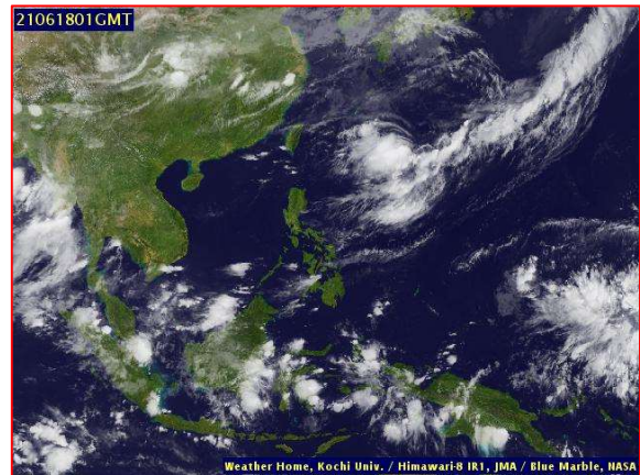
ภาพถ่ายดาวเทียม วันที่ ๑๘ มิ.ย. ๒๕๖๔ เวลา ๐๘.๐๐ น.
