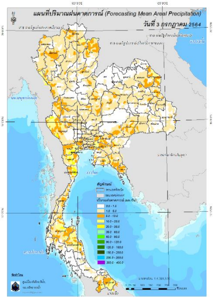
ปริมาณฝนคาดการณ์ในวันที่ 3 กรกฎาคม 2564
