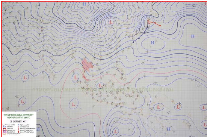
แผนที่อากาศ วันที่ ๑๙ ม.ค. ๒๕๖๐ เวลา ๐๖.๐๐ น.
