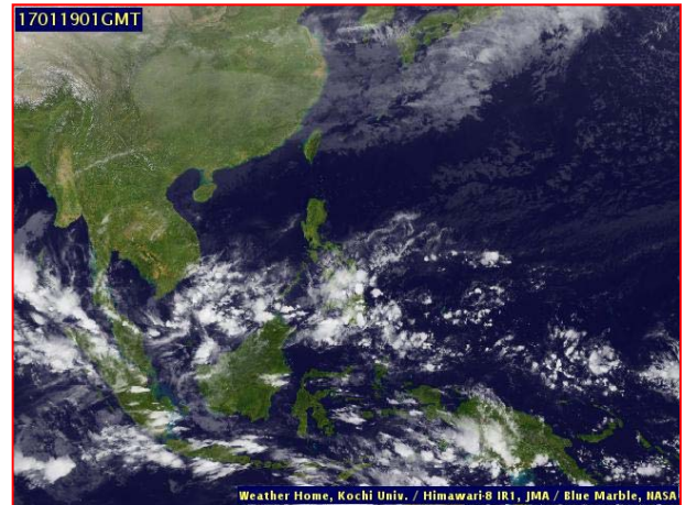
ภาพถ่ายจากดาวเทียม วันที่ ๑๙ ม.ค. ๒๕๖๐ เวลา ๐๘.๐๐ น.
