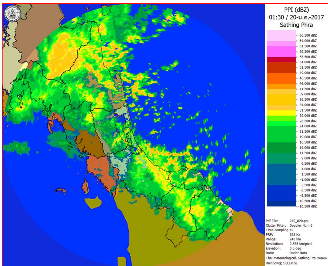
ภาพเรดาร์ตรวจอากาศ “สทิงพระ” ณ วันที่ 20 มกราคม 2560 (ที่มา : กรมอุตุนิยมวิทยา)
