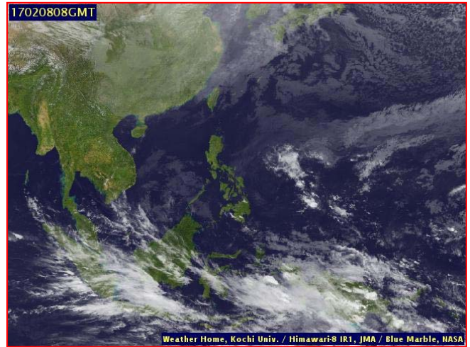
ภาพถ่ายจากดาวเทียม วันที่ ๘ ก.พ. ๒๕๖๐ เวลา ๑๕.๐๐ น.
