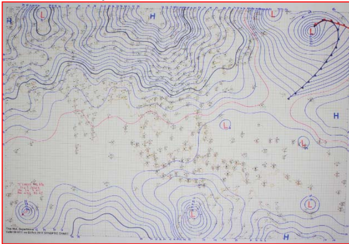
แผนที่อากาศ วันที่ ๘ ก.พ. ๒๕๖๐ เวลา ๐๗.๐๐ น.
