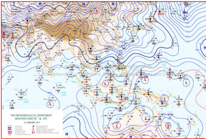
แผนที่อากาศ วันที่ ๑๔ ก.พ. ๒๕๖๐ เวลา ๐๑.๐๐ น.
