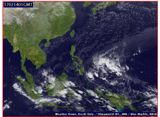
ภาพถ่ายจากดาวเทียม วันที่ ๑๔ ก.พ. ๒๕๖๐ เวลา ๐๗.๐๐ น.
