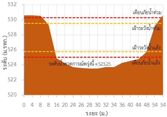
TC011008 สะพานบ้านคองฝ้าง - บ้านห้วยสิงห์
