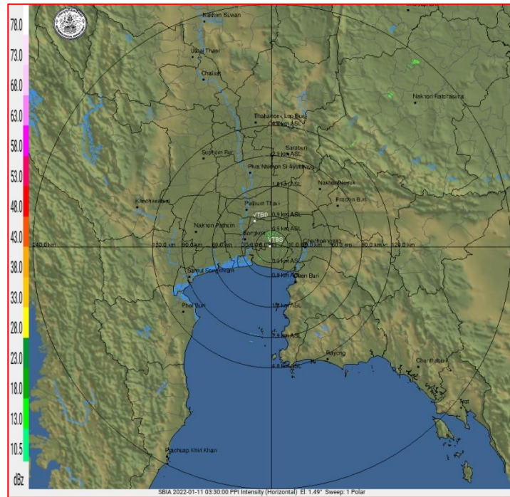
ภาพเรดาร์ตรวจอากาศ “สถานีสุวรรณภูมิ” ณ วันที่ 11 มกราคม 2565 เวลา 10.30 น. (ที่มา : กรมอุตุนิยมวิทยา)
