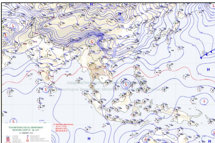
แผนที่อากาศ วันที่ ๒๘ ม.ค. ๒๕๖๕ เวลา ๐๑.๐๐ น.
