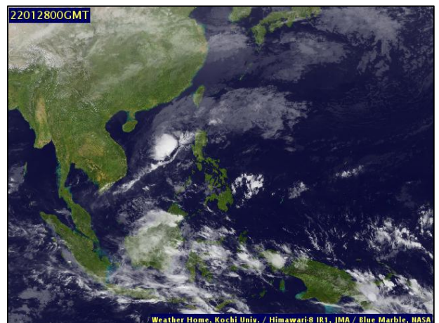
ภาพถ่ายดาวเทียม วันที่ ๒๘ ม.ค. ๒๕๖๕ เวลา ๐๗.๐๐ น.
