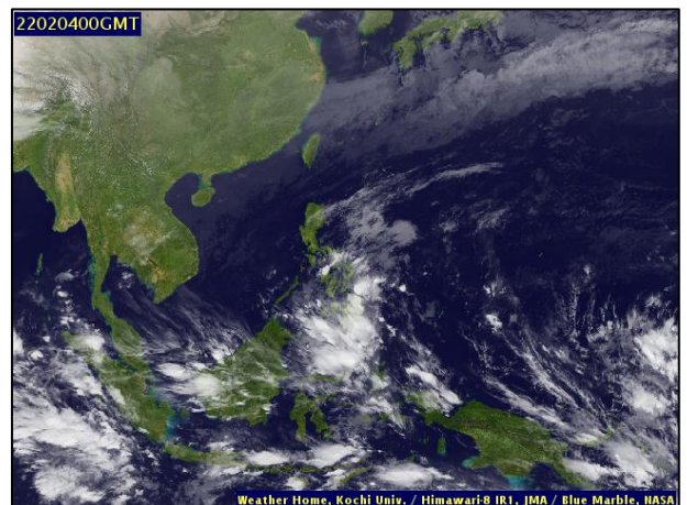
ภาพถ่ายดาวเทียม วันที่ ๔ ก.พ. ๒๕๖๕ เวลา ๐๗.๐๐ น.
