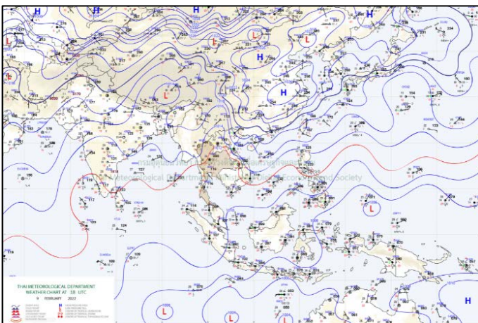
แผนที่อากาศ วันที่ ๑๐ ก.พ. ๒๕๖๕ เวลา ๐๑.๐๐ น.
