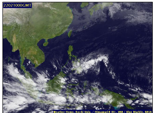
ภาพถ่ายดาวเทียม วันที่ ๑๐ ก.พ. ๒๕๖๕ เวลา ๐๗.๐๐ น.
