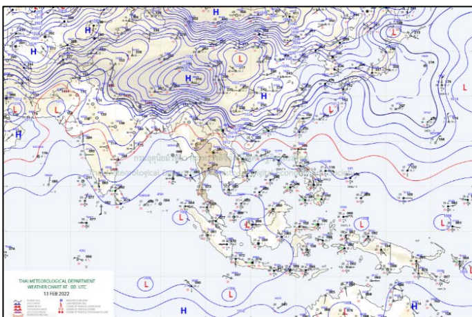
แผนที่อากาศ วันที่ ๑๓ ก.พ. ๒๕๖๕ เวลา ๐๗.๐๐ น.
