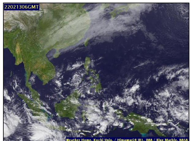
ภาพถ่ายดาวเทียม วันที่ ๑๓ ก.พ. ๒๕๖๕ เวลา ๑๓.๐๐ น.
