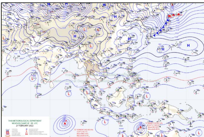
แผนที่อากาศ วันที่ ๒๗ ก.พ. ๒๕๖๕ เวลา ๐๗.๐๐ น.
