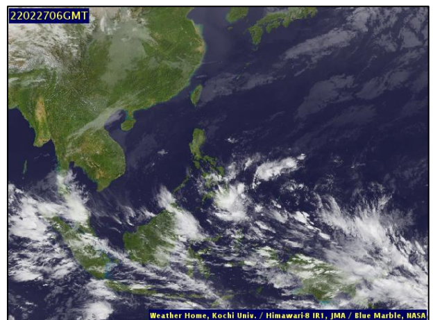
ภาพถ่ายดาวเทียม วันที่ ๒๗ ก.พ. ๒๕๖๕ เวลา ๑๓.๐๐ น.
