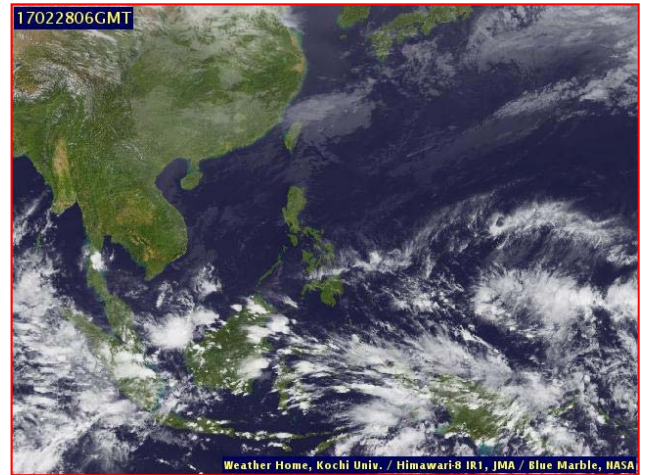
ภาพถ่ายจากดาวเทียม วันที่ ๒๘ ก.พ. ๒๕๖๐ เวลา ๑๓.๐๐ น.
