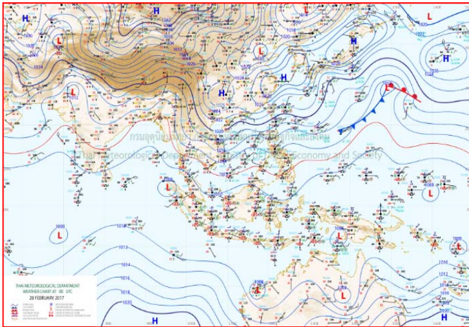
แผนที่อากาศ วันที่ ๒๘ ก.พ. ๒๕๖๐ เวลา ๐๗.๐๐ น.
