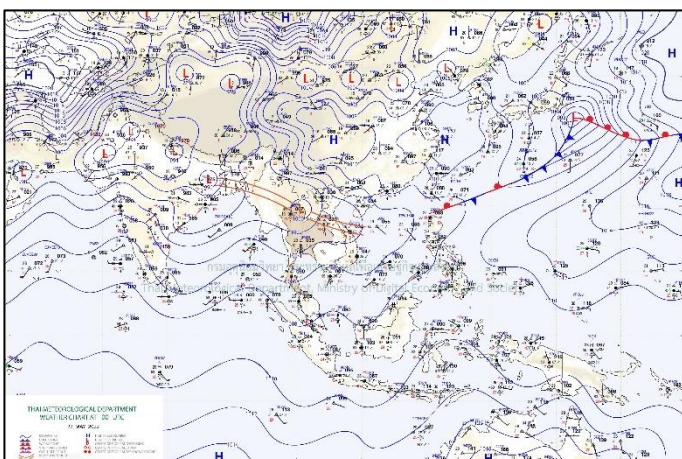
แผนที่อากาศ วันที่ ๒๒ พ.ค. ๒๕๖๕ เวลา ๐๗.๐๐ น.
