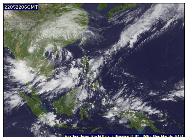
ภาพถ่ายดาวเทียม วันที่ ๒๒ พ.ค. ๒๕๖๕ เวลา ๑๓.๐๐ น.
