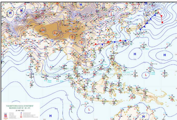
แผนที่อากาศ วันที่ ๒๙ พ.ค. ๒๕๖๕ เวลา ๐๑.๐๐ น.
