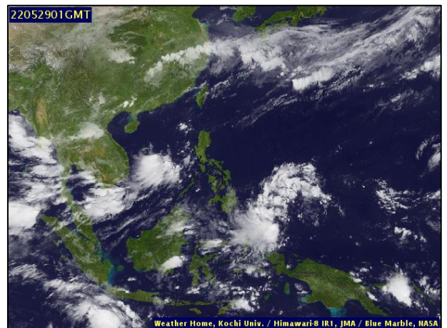
ภาพถ่ายดาวเทียม วันที่ ๒๙ พ.ค. ๒๕๖๕ เวลา ๐๗.๐๐ น.
