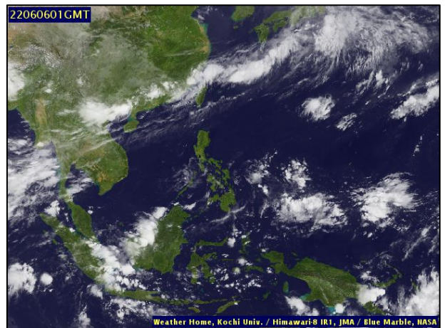
ภาพถ่ายดาวเทียม วันที่ ๖ มิ.ย. ๒๕๖๕ เวลา ๐๘.๐๐ น.
