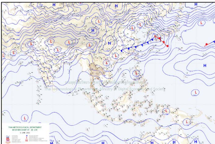
แผนที่อากาศ วันที่ ๖ มิ.ย. ๒๕๖๕ เวลา ๐๑.๐๐ น.
