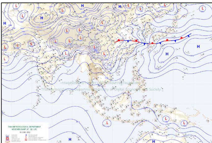
แผนที่อากาศ วันที่ ๑๙ มิ.ย. ๒๕๖๕ เวลา ๐๑.๐๐ น.
