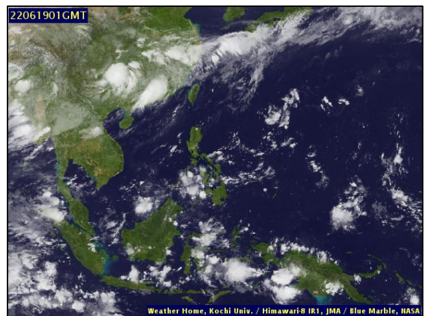
ภาพถ่ายดาวเทียม วันที่ ๑๙ มิ.ย. ๒๕๖๕ เวลา ๐๘.๐๐ น.
