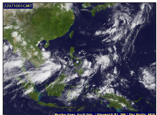
ภาพถ่ายดาวเทียม วันที่ ๑๐ ก.ค. ๒๕๖๕ เวลา ๐๘.๐๐ น.
