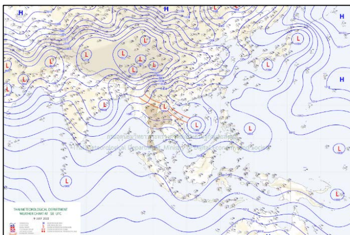
แผนที่อากาศ วันที่ ๑๐ ก.ค. ๒๕๖๕ เวลา ๐๑.๐๐ น.
