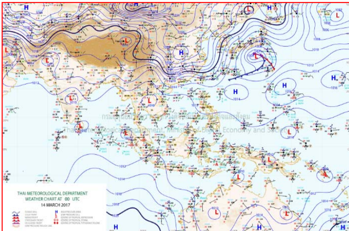
แผนที่อากาศ วันที่ ๑๔ มี.ค. ๒๕๖๐ เวลา ๐๗.๐๐ น.
