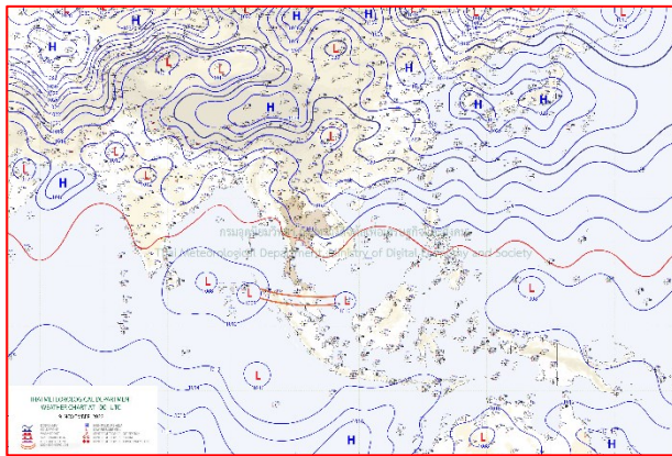
แผนที่อากาศ วันที่ 9 พ.ย. 2565 เวลา 07.00 น.
