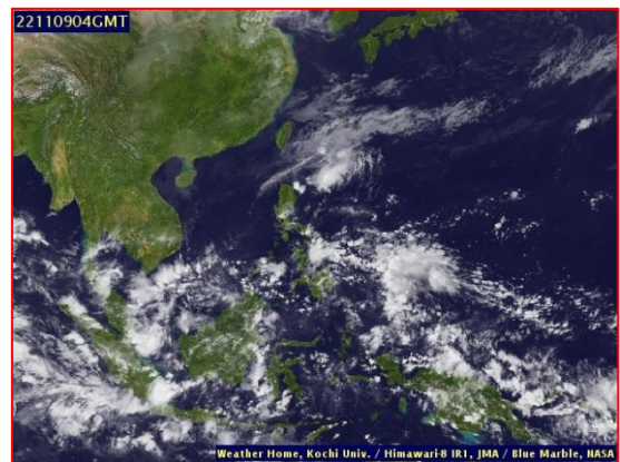
ภาพถ่ายจากดาวเทียม วันที่ 9 พ.ย. 2565
